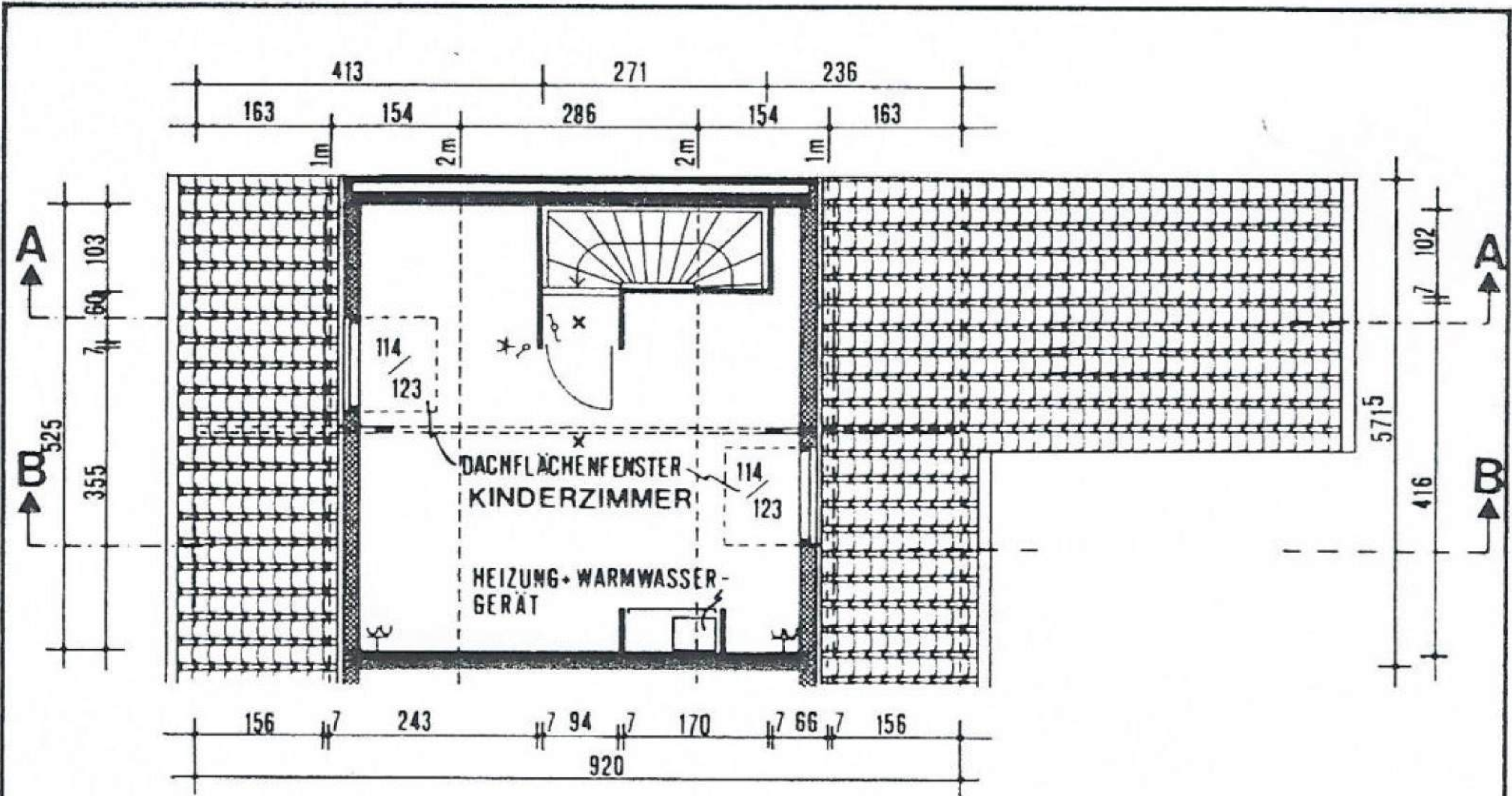
DACHGESCHOSS
